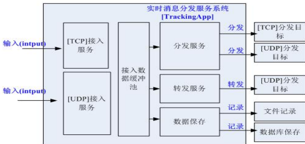
实时消息分发服务系统平台流程图：
